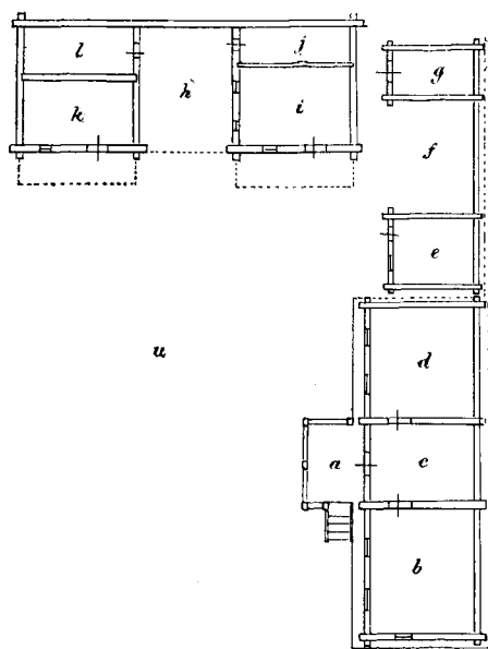
Planul casei și al celorlalte clădiri economice.) a) privariu; b) casa cea mare; c) tindă; d) coamăr; e) căsoaie; f) șopru; g) latrină; h) aria șurii; i) grajd; j. grăjdet (pleșnicar); k) grajd de bucate; l) grăjdet; m) curte
