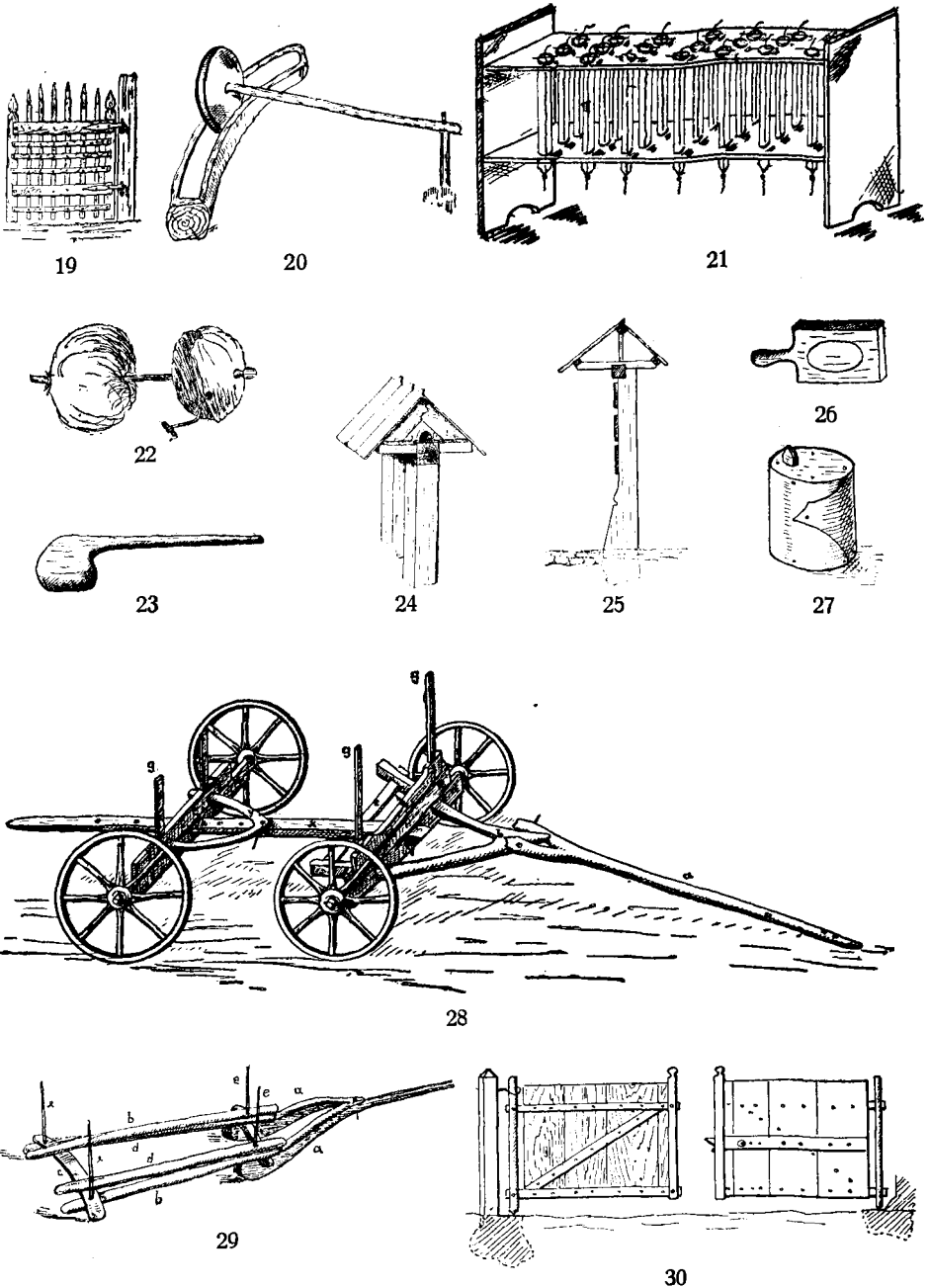
Fig. 19. Ușița dela gărlciu; 20. Pisătoare de mere; 21. Scaun de lumânări; 22. Sfărăitoare; 23. Maiu; 24—25. Coperișul porțiței; 26. Blăniță de tocat carne; 27. Solniță; 28. Carul de lemne: a) hoîștea, b) pisc, c) brăcinar, d) osia dinainte, e) pod, f) fercheteu, g) mânuși, h) cuiul inimii, i) osia dinapoi, x) inima, y) gemânare; 29. Scîlifa: a) sanie, b) tălpi, c) oplean, d) prăjini, e) mânuși; 30. Porțiță.
