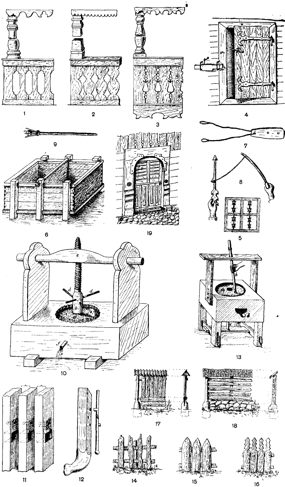
Fig. 1—3 Detalii de privariu; 4. ușa dela coamăr; 5. fereastră; 6. coș de bucate; 7. sbârnaitoare; 8. săgeată; 9. praștie; 10. teasc; 11—12 încuietoare de lemn; 13. rășniță; 14—18 îngrădituri.
