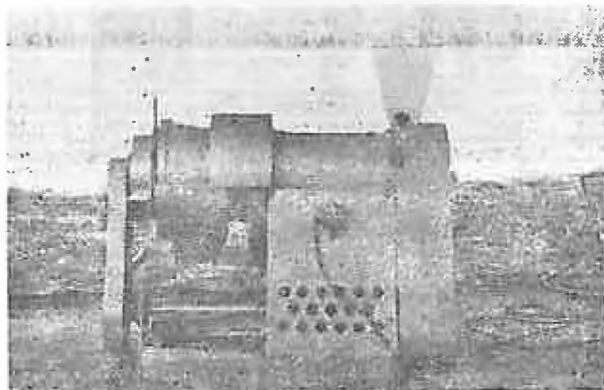
Fig. 16. Mașina de dezariptat semințe de pini și molii.
