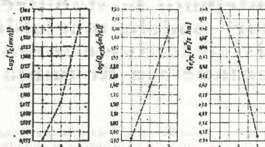
Fig. 2. Modele hidrologice ale unui bazin torențial montan din România situat în arealul sisturilor cristaline (Bazinul Bîrsa superioară). a) Timpul de concentrare a scurgerii în bazin; b) Debitul maxim de viitură „morfo-etalon”; c) Debitul specific maxim de viitură „morfo-etalon”; 1...3 — Ordinele hidrografice.
