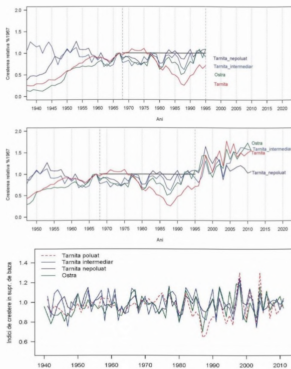
Fig. 4. Serii de indici. Calculul, analiza și evoluția indicilor de creștere calculați în raport cu suprafața de bază în suprafețele de probă Tarnița nepoluată, Tarnița intermediară, Tarnița (poluat) și Ostra
