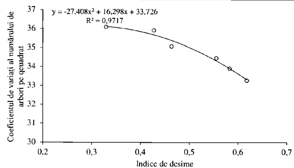
Fig. 3. Relația dintre indicele de desime și coeficientul de variație al numărului mediu de arbori pe quadrat.
