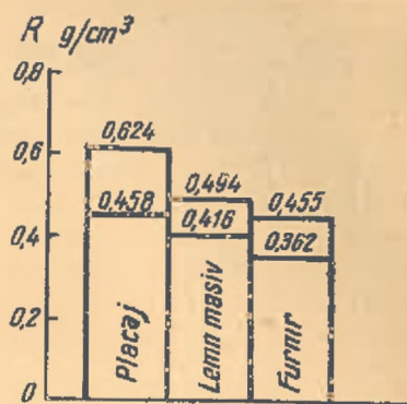
Fig. 3. — Densitatea „R” a placajelor, furnirilor și lemnului masiv (valori maxime și minime)
