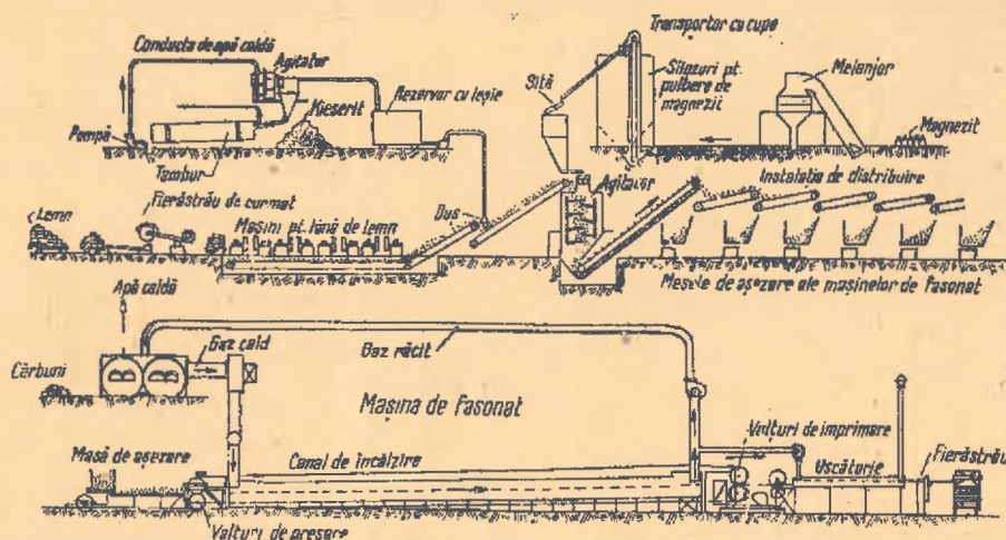
Fig. 2. Schema fabricării plăcilor din lână de lemn prin procedeul Heraklith.
