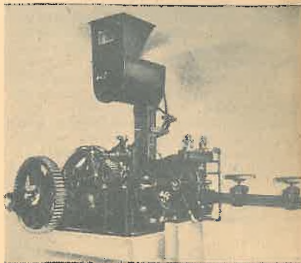
Fig. 23. Instalație pentru brichetat rumegușul.
