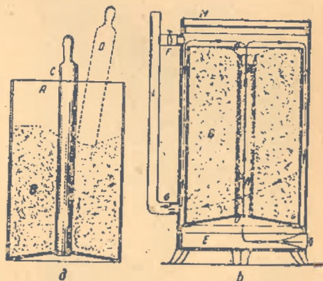
Fig. 14. Schema unei sobe pentru rumeguș: A—cutie metalică („garnitură”) pentru încărcat rumegușul, B—încărcătura de rumeguș, C—cilindru de lemn, D—maiu de lemn pentru bătut rumegușul, E—cutie pentru cenușe, F—clapă pentru reglarea tirajului, G—deschiderea spre coș, H—capac, K—canal de ardere, L—burlan, O—deschiderea de jos.
