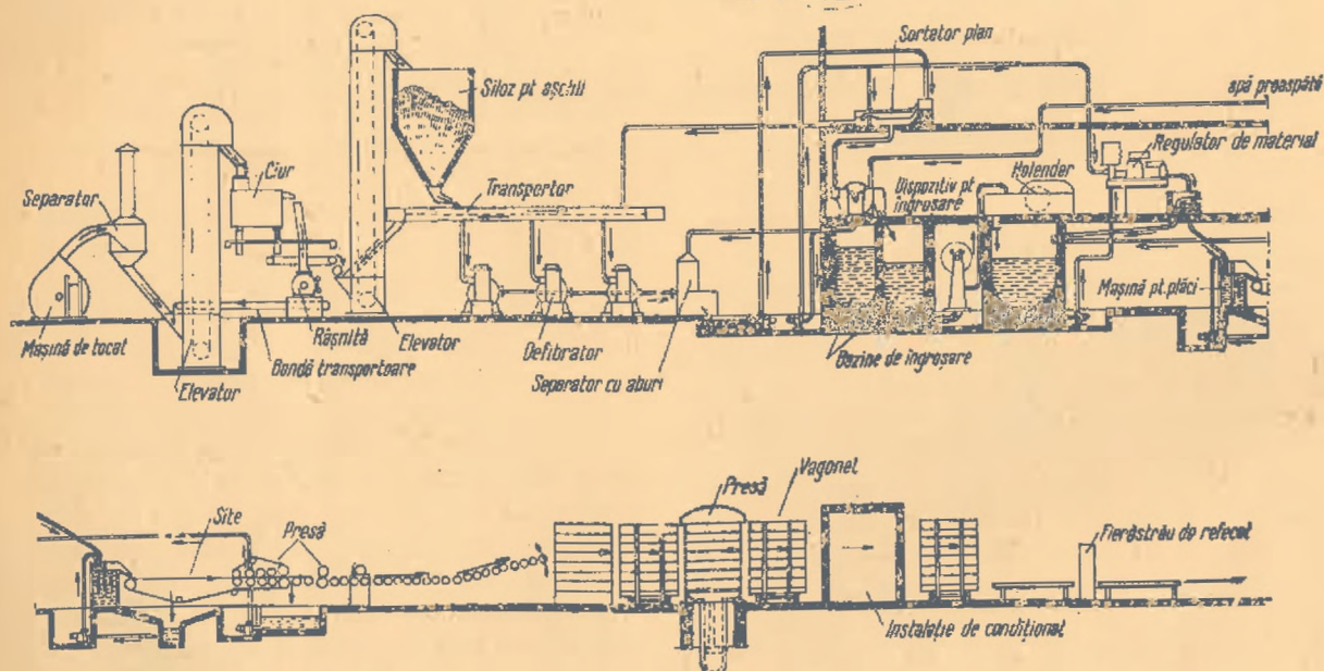
Fig. 5. Schema fabricării plăcilor din fibre de lemn prin procedeul „defibrator”.
