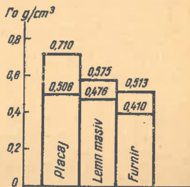
Fig. 4. — Densitatea „r0” a placajelor, furnirilor și lemnului masiv (valori maxime și minime)
