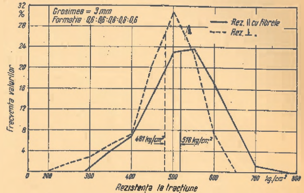
Fig. 6. — Curbele de frecvență a valorilor rezistenței la tracțiune a plăcajelor de anin.
