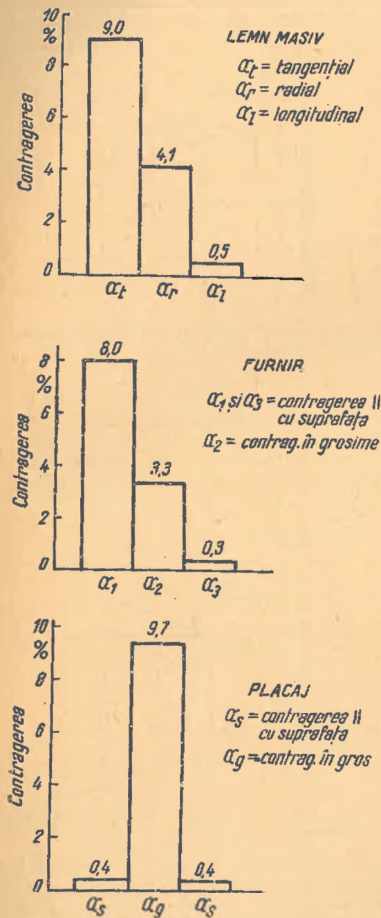
Fig. 5. — Contragerea totală a lemnului masiv, furnirelor și placajelor de anin (valori mijlocii).
