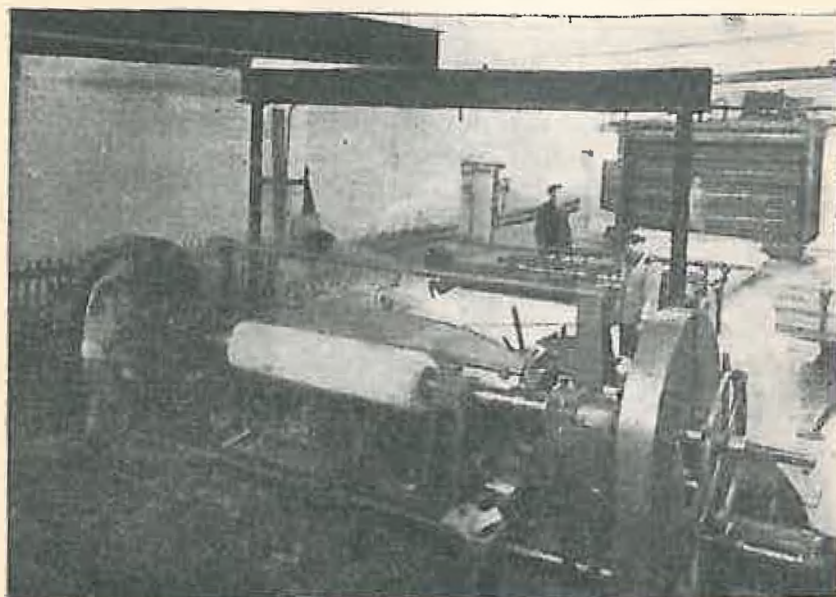
Fig. 2. — O mașină de derulat furnir văzută din spate. (După Knight-Wulpi: Furniere und Sperrholz, Bd. I. 1930). Banda de furnir merge direct la foarfecile de tăiat.
