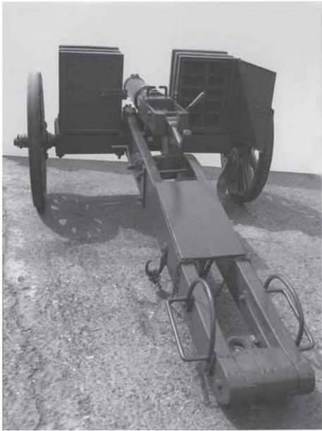
■ Prima armă automată din dotarea armatei române, mitraliera Christopher & Montigny, md. 1872
