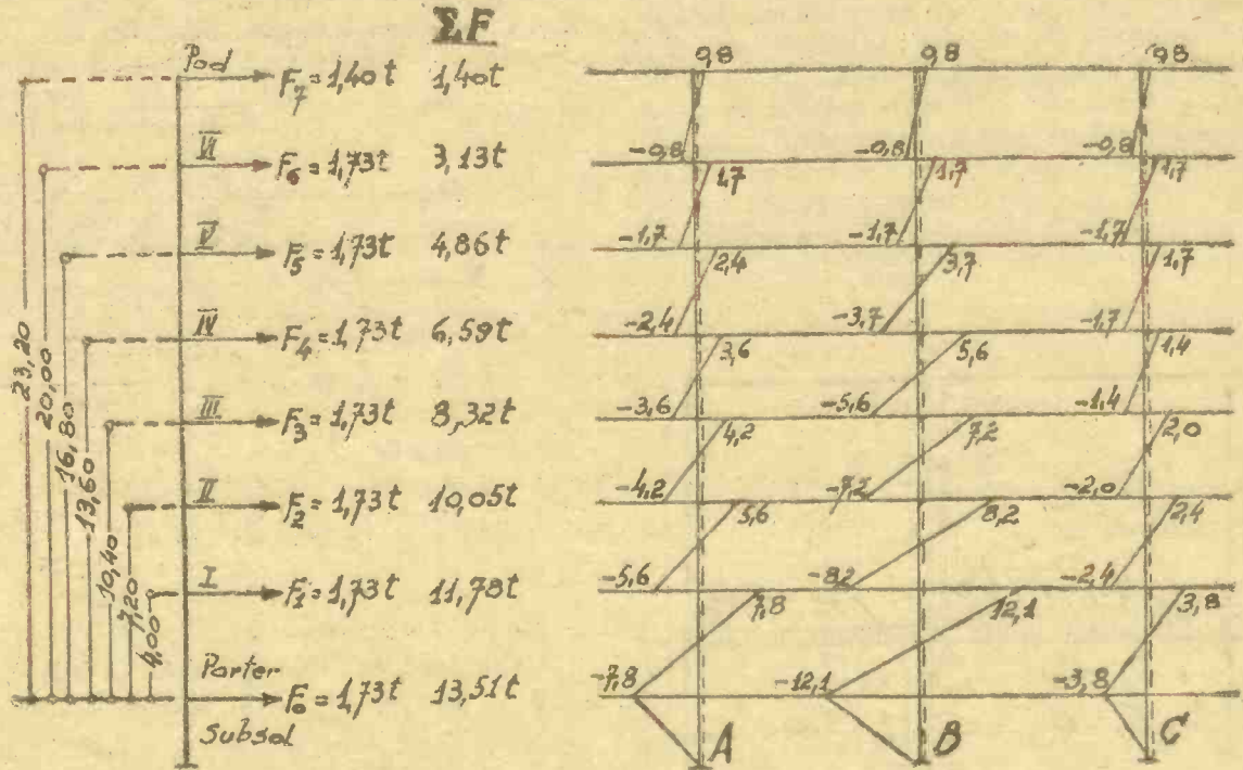
Diagrama momentelor încovoetoare în stâlpi:
