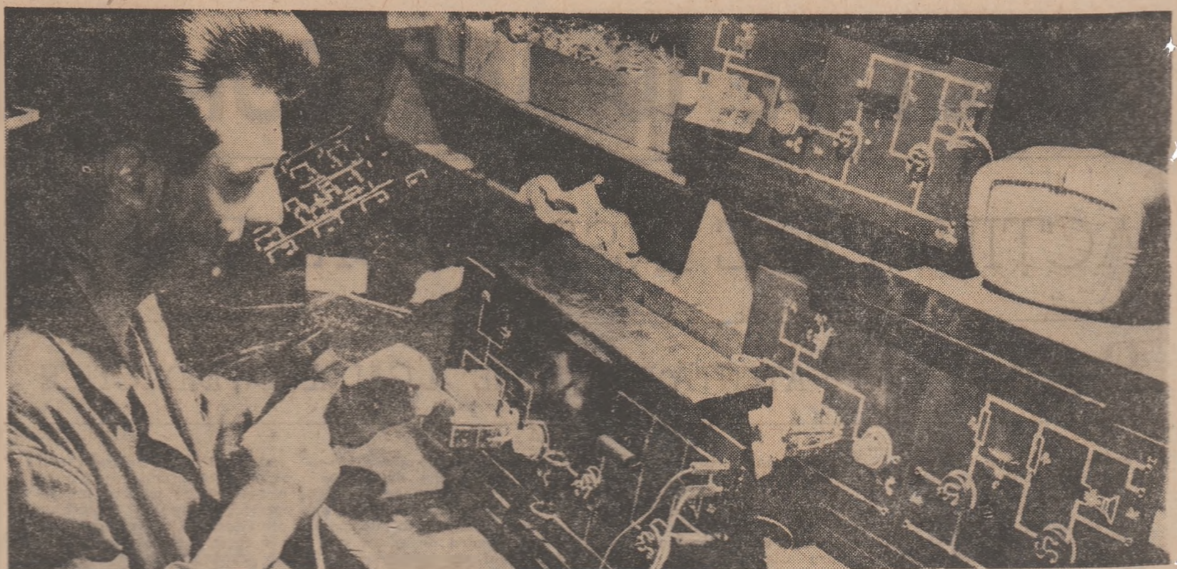
Truse electronice cu semiconductori, produse de I.M.D., pentru predarea noțiunilor de electromagnetism
