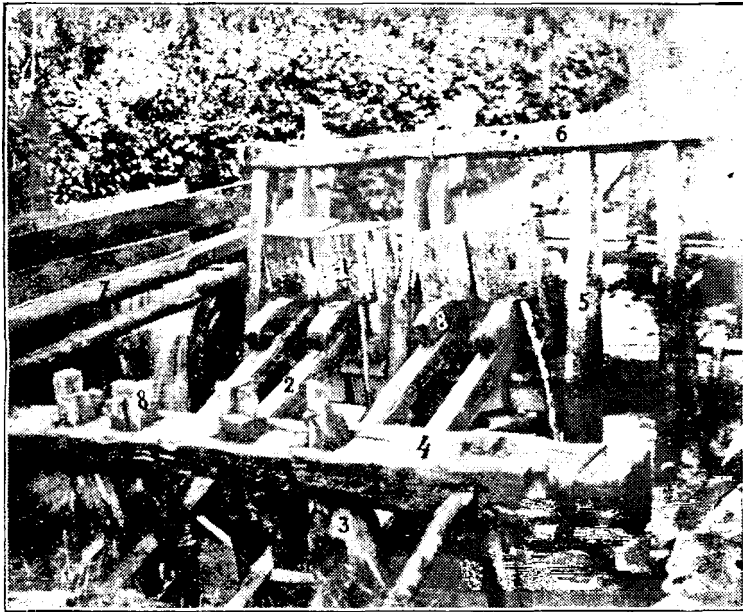
Vederea piuălor. 1. Pilug; 2. Tânel; 3. Urs; 4. Grinda dinapoi (a urșilor); 5. Spătare; 6. Grinda piuălor; 7. Cioroiu; 8. Ieuri (găvoazde). (Foto I. Morariu)
