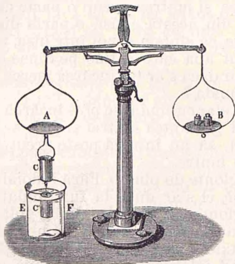
Balanță care arată că un corp cufundat în apă pierde din greutate.
