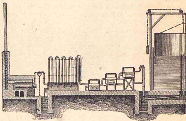
Fig. 3. Fabricarea gazului de iluminat din cărbunii de pământ.
