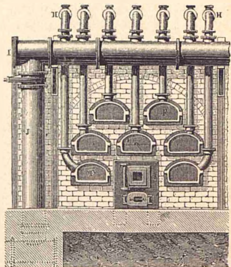
Fig. 2. Furnalul și cilindrele de gresie ale usinei de gaz.
