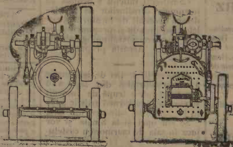
LOCOMOBILA LEMAITRE
