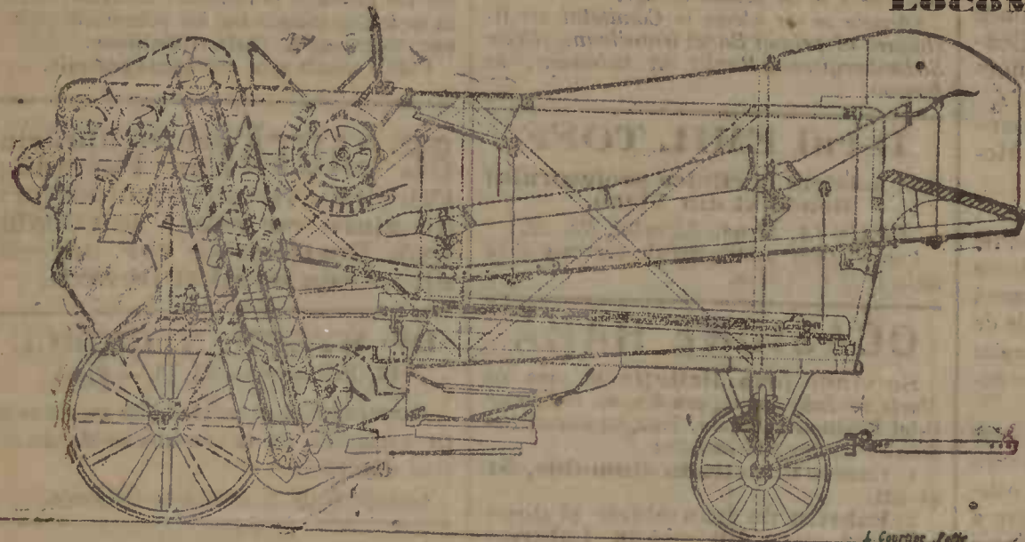
BATOZA „LEMAITRE“
