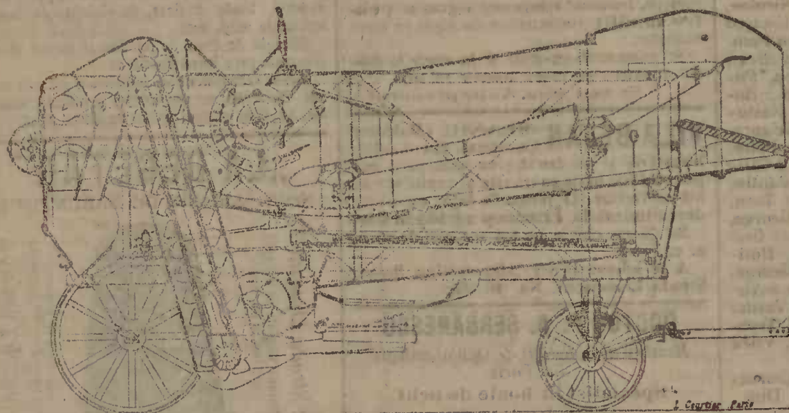
BATOZA „LEMAÎTRE“
