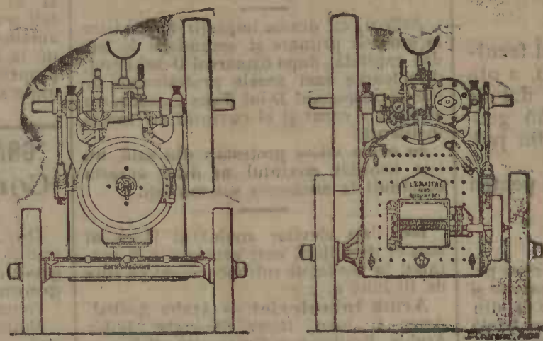
LOCOMOBILA LEMAÎTRE
