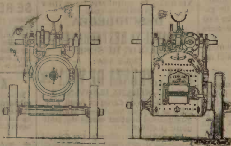
LOCOMOBILA LEMAITRE
