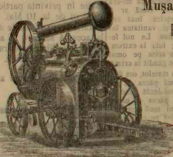
Locomobilă cu aparat de ars pae automatice
