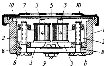
Capsulă telefonică
