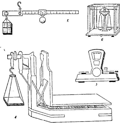
Balanțe: 1 — balanță romană; 2 — balanță analitică; 3 — balanță Roberval; 4 — balanță zecimală
