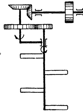
Agitator (2)
