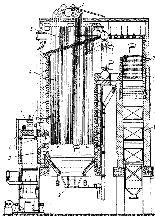
Cazan cu țevi de apă
