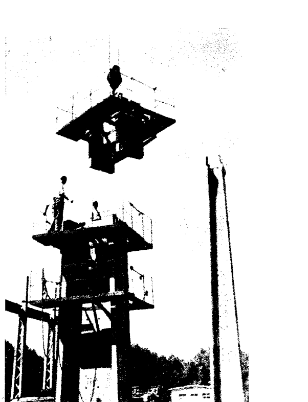
Stilpi pentru cale de rulare exterioară, executați din boltari asamblați prin precomprimare la Uzinele chimice Făgăraș
