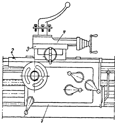
Cărucior de strung
