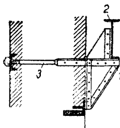
Consolă de perete pentru pod rulant: 1 — consolă; 2 — grindă de rulare; 3 — ancoraj.
