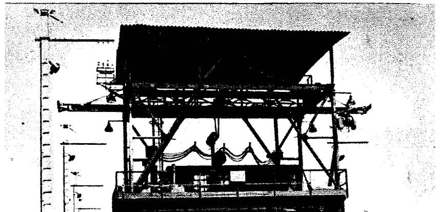
Întreprinderea de prefabricate „Progresul” București Linie tehnologică pentru fișii de planșee
