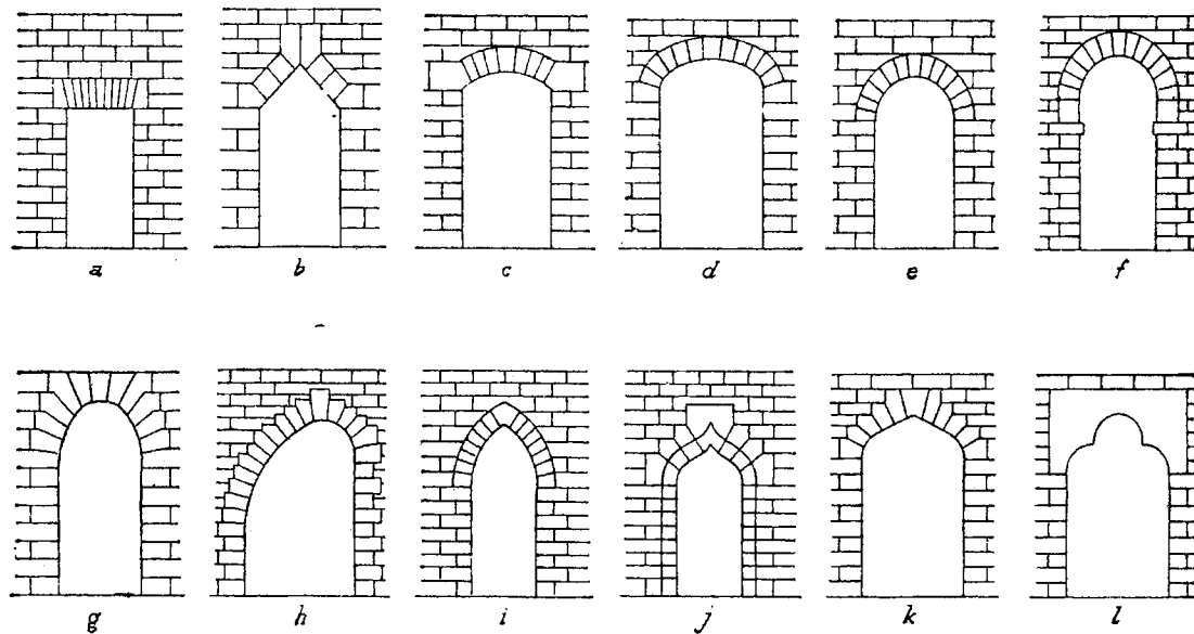
Arc a — arc plat; b — arc în unghi ascuțit; c — arc bombat; d — arc în mîner de coș; e — arc în plin cintru; f — arc suprainălțat; g — arc eliptic; h — arc rampant; i — arc în ogivă; j — arc în acoladă; k — arc Tudor; l — arc trilobat
