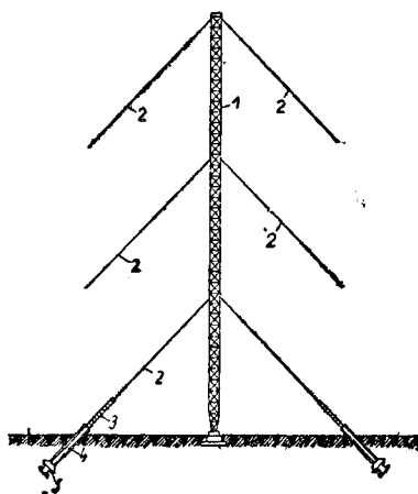
Ancorarea unui pilon metalic de antenă de radioemisiune
