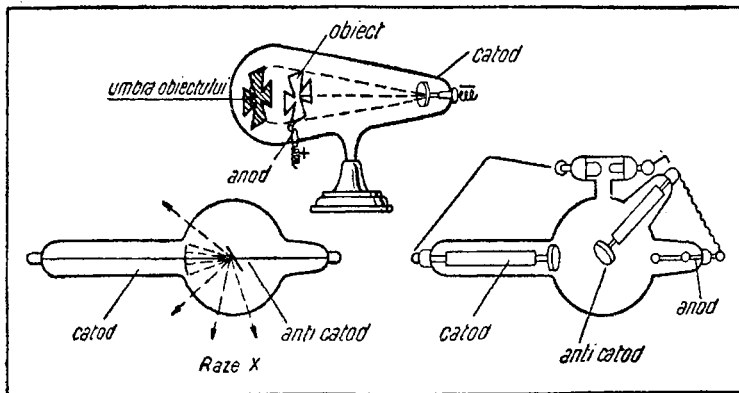
Diverse tipuri de tuburi Crookes
