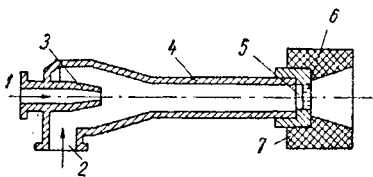
Arzător
