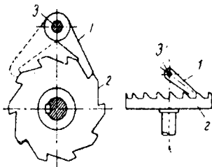
Clichet de blocare 1 — clichet; 2 — roată înclichetabilă; 3 — axul clichetului
