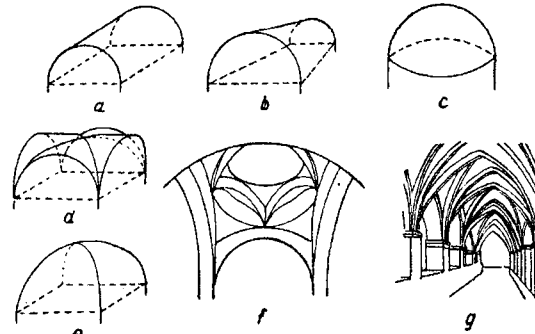
Tipuri de bolți
