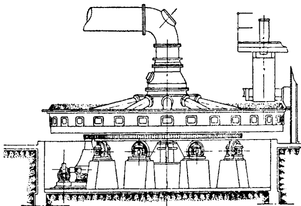
Agglomerator
