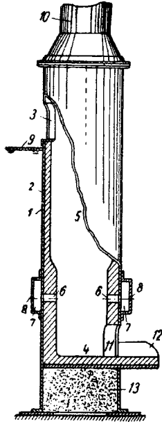
Cubilou
