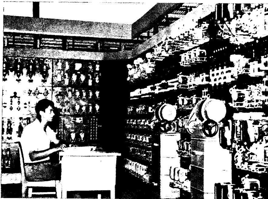
Stația aparaturii automate a furnalului de 700 m 3 de la Combinatul siderurgic Hunedoara.
