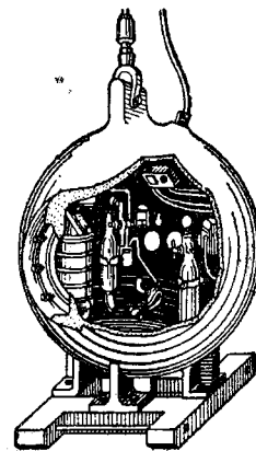
Batisferă
