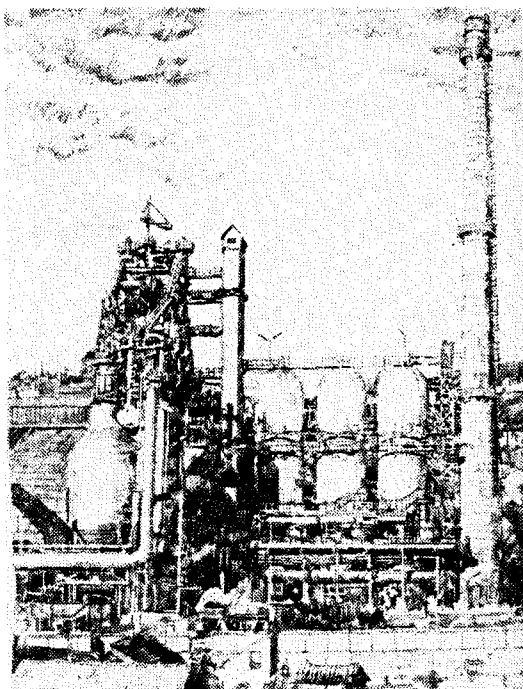
Furnalul de 700 m 3 de la Reșița
