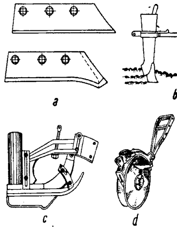
Brăzdare
