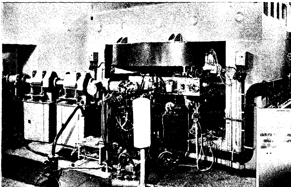
Ciclotronul I.F.A. (R.P.R.)
