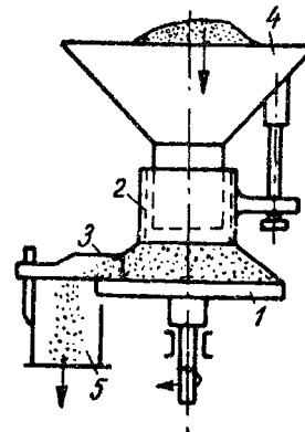
Alimentator
