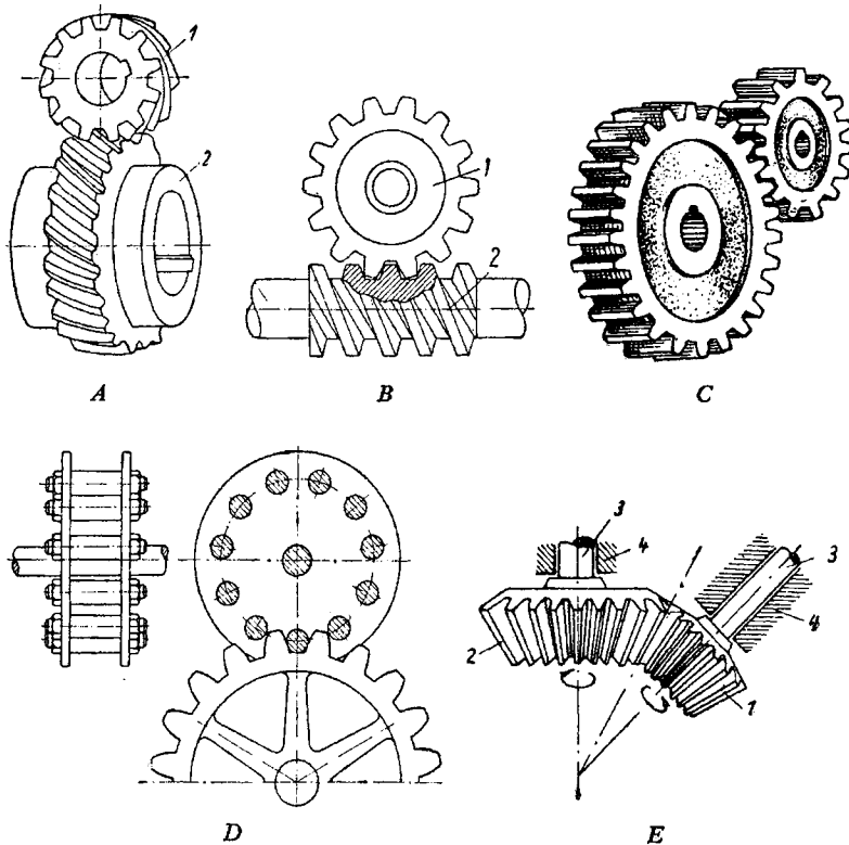
A. Angrenaj elicoidal: 1 — roată conducătoare; 2 — roată condusă. B. Angrenaj cu melc: 1 — roată melcată; 2 — melc. C. Angrenaj cilindric. D. Angrenaj cu bolțuri. E. Angrenaj conic: 1 — roată conducătoare; 2 — roată condusă; 3 — arbore; 4 — palier.
