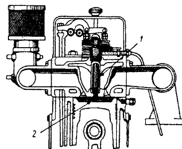
Camera de ardere a unui motor diesel 1 — injector de combustibil 2 — cameră de ardere
