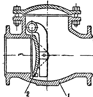
Robinet cu clapă de reținere
