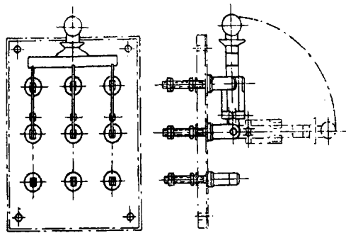
Comutator tripolar cu pîrghie
