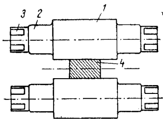
Cilindri de laminor
