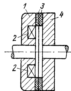
Ambreiāj electromagnetic 1—miez feromagnetic; 2—înfășurare; 3—suprafață de frecare; 4—armătură
