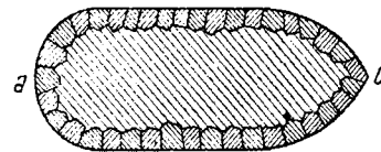
Secțiune transversală printr-o pilă de pod a — avanbec; b — arierbec
