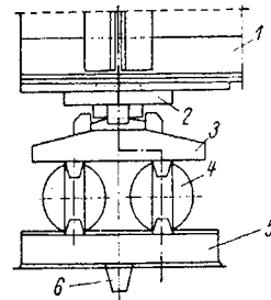
Aparat de reazem mobil cu balansiere 1 – grindă; 2 – balansiér superior; 3 – balansiér inferior; 4 – rulouri; 5 – placă de reazem; 6 – nervură
