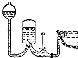
Berbec hidraulic
