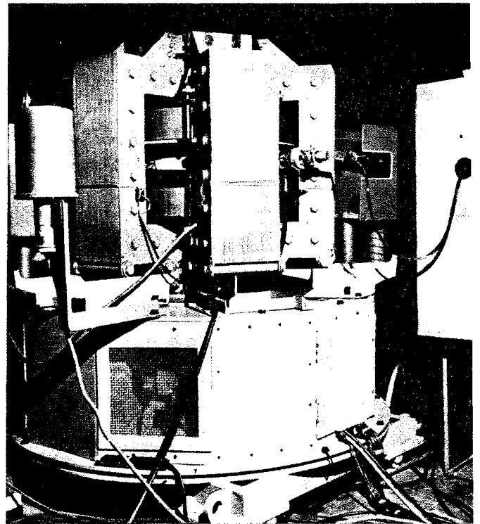
Betatronul I.F.A. (R.P.R.)
