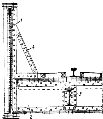
Pod metalic cu calea jos (jumătate de secțiune transversală a suprastructurii) 1 — grindă principală; 2 — antretoază; 3 — lonjeron; 4 — ranfort
