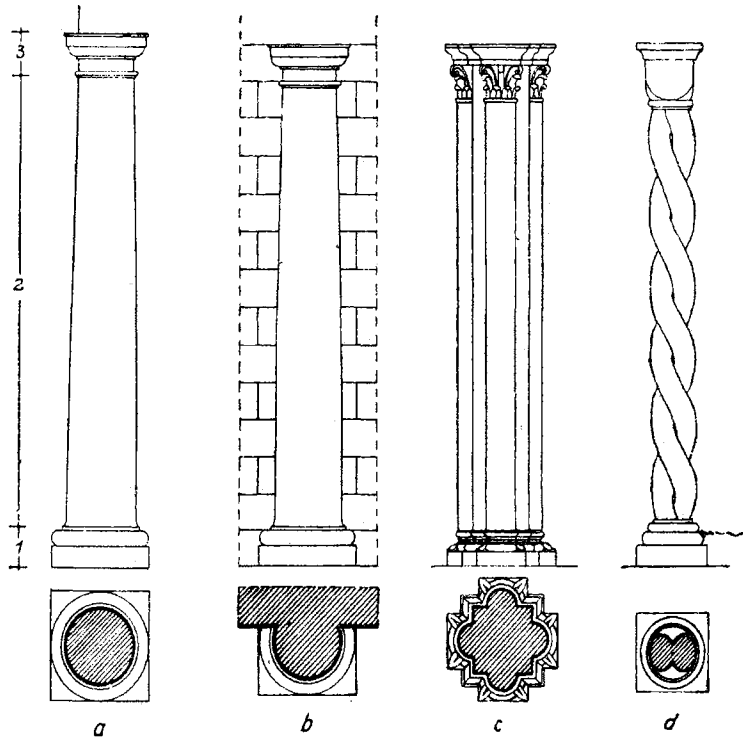
Tipuri de coloane
