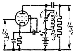
Amplificator
