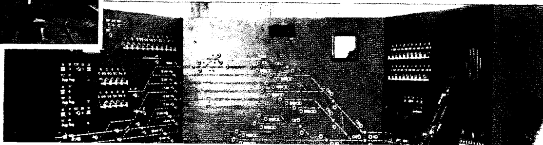
Panoul aparaturii de comandă automată pentru instalația de călire cu curenți de înaltă frecvență tip M.U.R. (R.P.R.)
