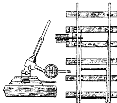
Ac de macaz
