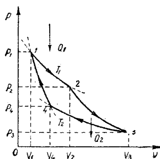
Ciclul lui Carnot
