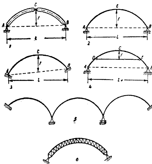
Tipuri de arcuri: 1 — arc cu trei articulații cu inimă plină (elementele componente); 2 — arc cu două articulații; 3 — arc încastrat; 4 — arc cu tirant; 5 — arc continuu; 6 — arc cu zăbrele. ABC — axa arcului; AB — linia nașterilor; A și B — nașteri C — cheia, f — săgeată; l — deschidere
