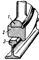
Bandaj 1 — discul roții; 2 — bandaj; 3 — șină
