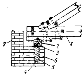
Rezemarea pe zid a babelor pentru ferme de acoperiș
