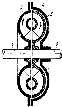
Ambreiaj hidraulic 1 — arbore antrenant; 2 — arbore antrenat; 3 — rotorul pompei; 4 — rotorul turbinei; 5 — carcasă
