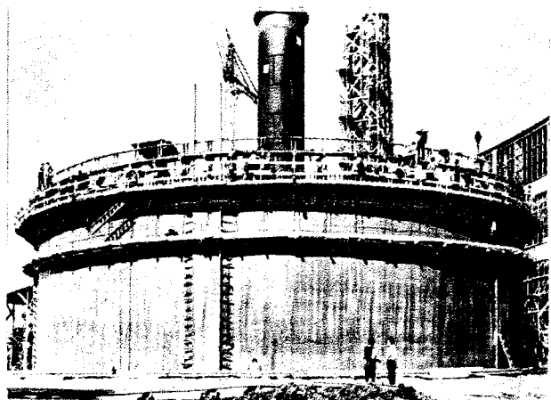
Siloz pentru zahăr din beton precomprimat, executat cu cofraje glisante, la fabrica „Siretul” Bucecea
