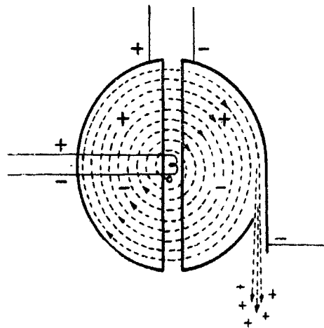
Schema de funcționare a ciclotronului
