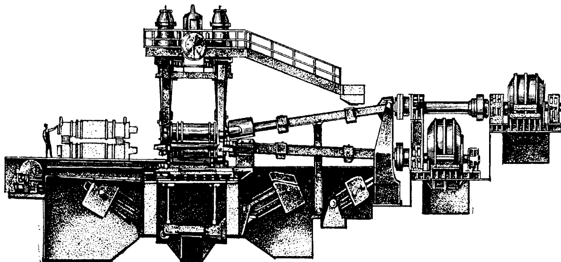
Linia principală a blumingului de 1150 mm.
