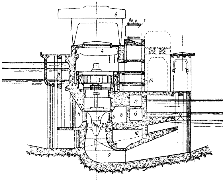
Secțiune printr-o centrală hidroelectrică
