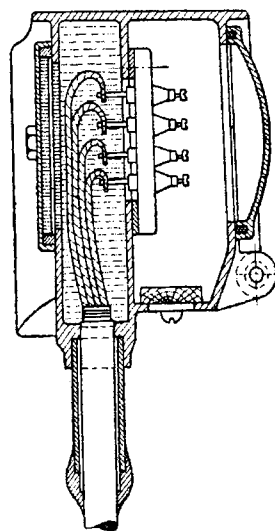
Cutie terminală
