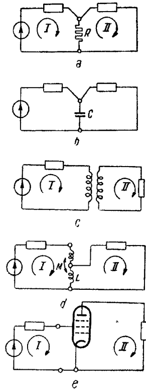
Cuplaj
