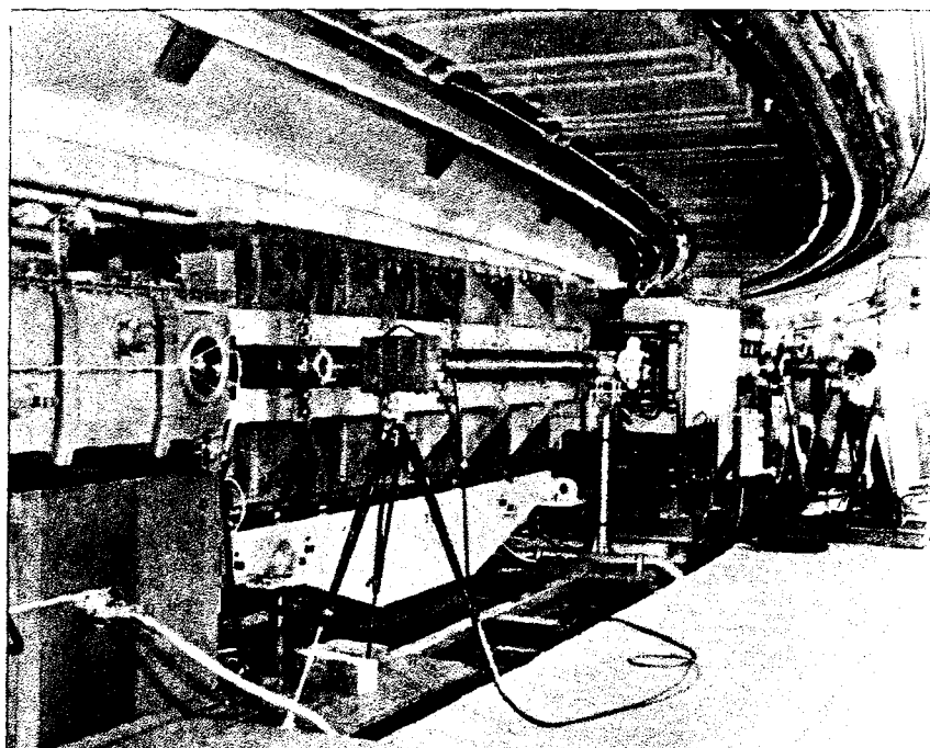
Ciclotronul I.F.A. (R.P.R.)
