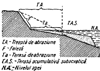
Abraziune (2)
