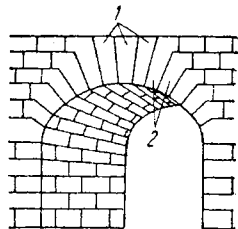
Bolț de piatră de talie 1 — bolțari obișnuiți; 2 — bolțari speciali
