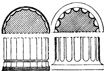
Caneluri (2)
