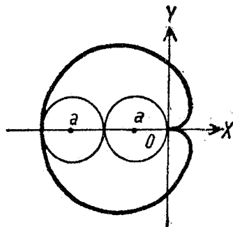
Cardioidă a — raza cercului
