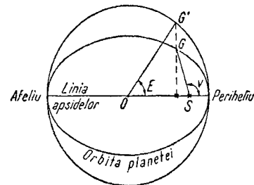
V — Anomalie adevărată; E — Anomalie excentrică
