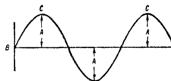
Amplitudine
