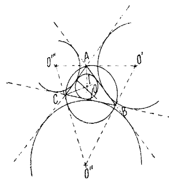
I — cerc circumscris; O — cerc înscris; O' , O'' , O''' — cercuri exînscrișe
