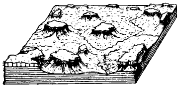
Bloctiagramă
