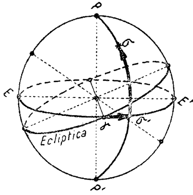
Coordonate ecuatoriale \gamma\sigma' — ascensiune dreaptă \sigma\sigma' — declinația \gamma — punctul vernal EE' — ecuatorul ceresc
