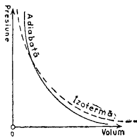
Adiabată
