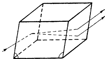
Birefringénță
