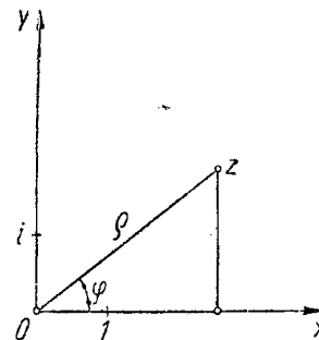
Argument (b)
