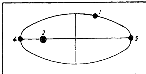
Apside
