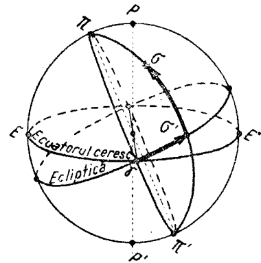
Coordonate ecliptice \gamma\sigma' — longitudinea cerească \gamma — punctul vernal \sigma\sigma' — latitudinea cerească \pi'\pi — polii eclipticii
