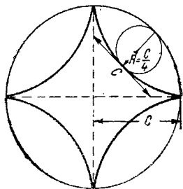
Astroidă
