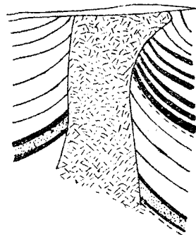
Cută diapiră
