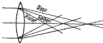
Aberație cromatică
