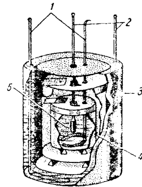
Calorimétru
