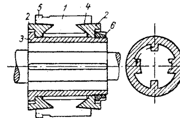
Colector de mașină electrică
