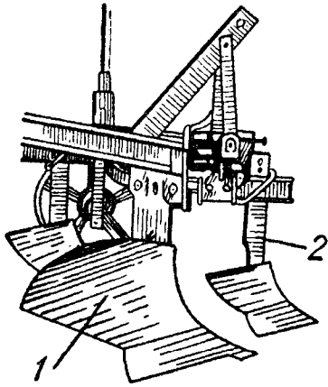
Plug cu antetrupiță 1 - Trupiță; 2 - Antetrupiță
