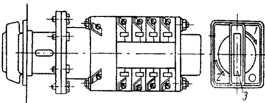
Comutator de comandă rotativ
