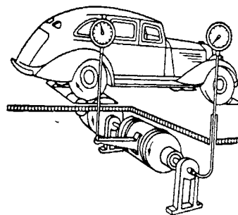
Banc de probă
