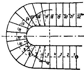
Balansarea treptelor unei scări, după metoda semicercului (construcție grafică în plan)
