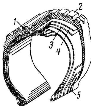
Anvelopă
