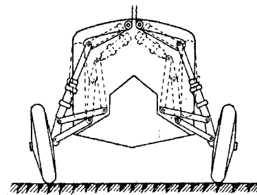
Aterizor
