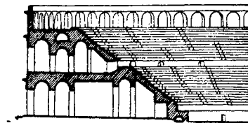
Amfiteatru. Secțiune
