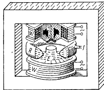
Schiță simplificată a betatronului R – tub de accelerare; W – bobine de magnetizare; E – fascicul de electroni P – piesă polară
