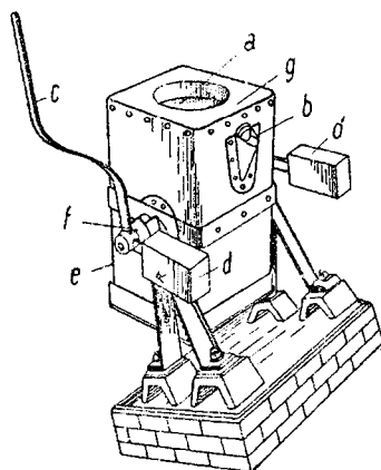
Cuptor cu creuzet
