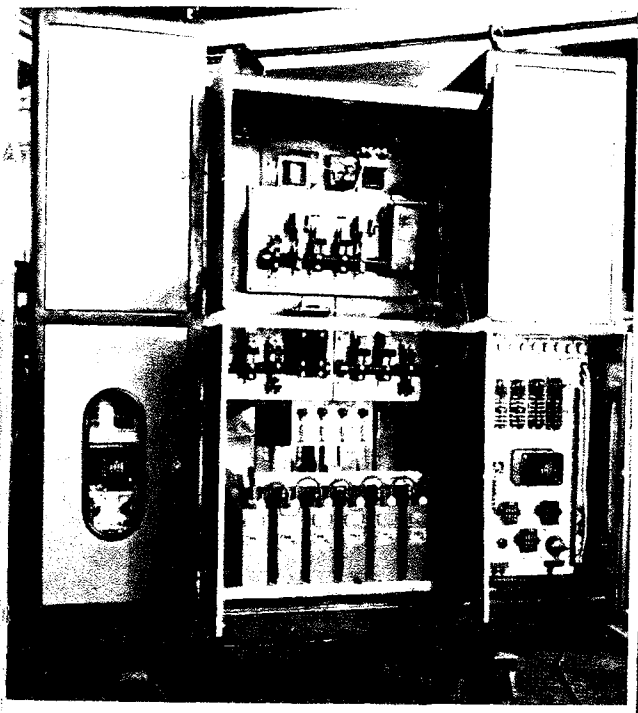
Panoul aparaturii de comandă automată pentru instalația de călire cu curenți de înaltă frecvență tip M.U.R. (R.P.R.)
