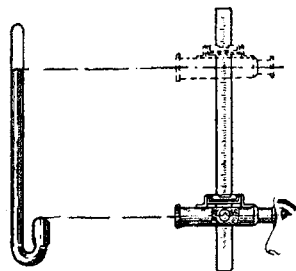
Catetometru
