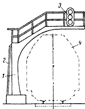
Consolă de semnal: 1 — consolă; 2 — scară de acces; 3 — semnal optic; 4 — gabarit de liberă trecere
