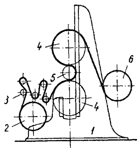
Calandru cu trei cilindre 1 — batiu; 2 — suportul sulului alimentator; 3 — role de conducere; 4 — cilindru elastic de presiune; 5 — cilindru metalic încălzit; 6 — suportul sulului înfășurător
