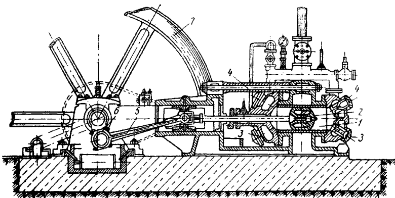
Compresor
