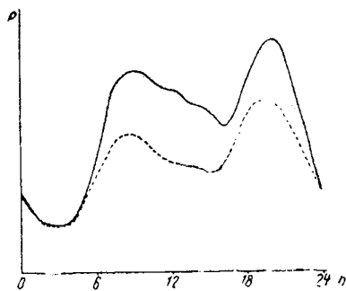
Curba de sarcină medie pentru o zi lucrătoare (linia continuă) și pentru o zi de sâmbătoare (linia întreruptă)
