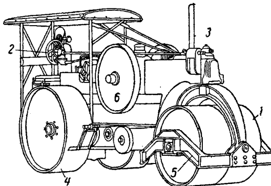
Compresor rutier
