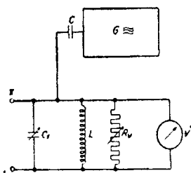
Admitanțmetru
