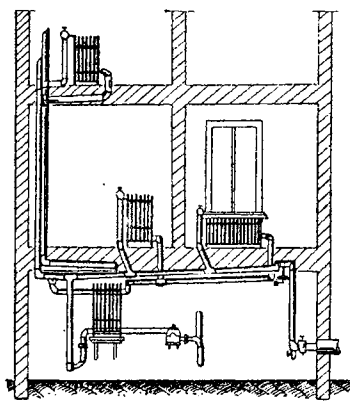
Calorifer
