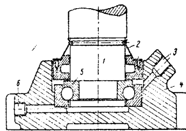
Crapodină
