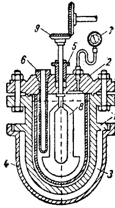
Autoclavă cu agitator
