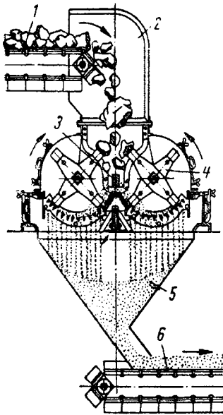
Concasor cu ciocane
