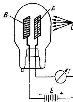
Celulă fotoelectrică
