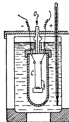
Bombă calorimetrică C — electrozi; O 2 — oxigen
