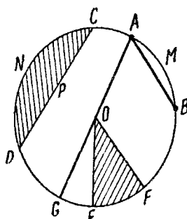
Cerc
