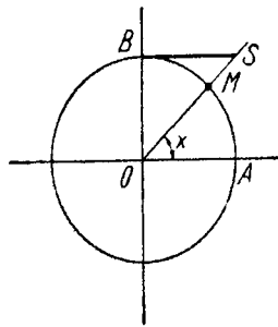
BS — cotangentă
