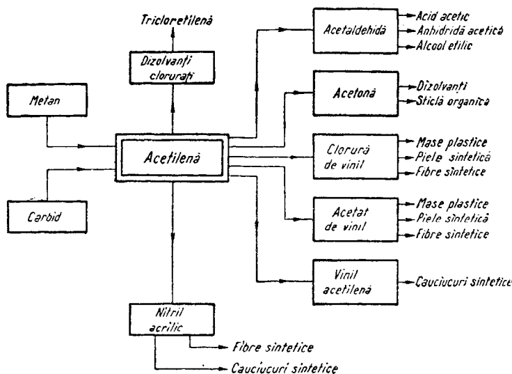
Obținerea acetilenei și domeniile mai importante de utilizare a ei
