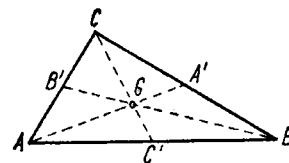
Baricentru
