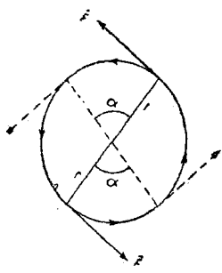
Cuplu de forțe
