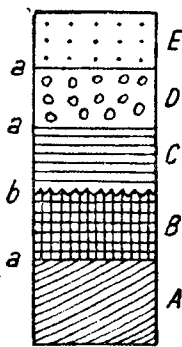
Coloană stratigrafică
