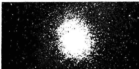
Roi de stele globular din constelația Hercule
