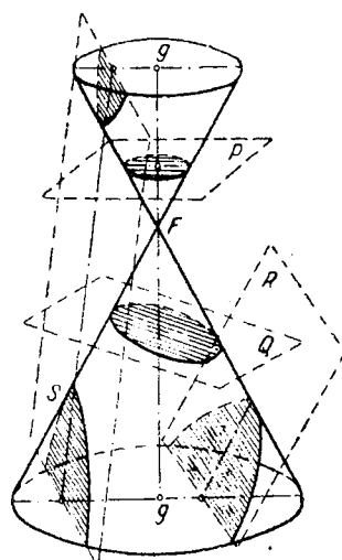
Conică
