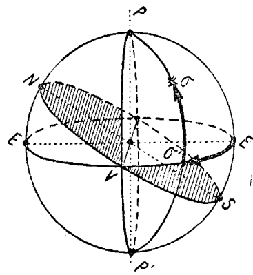
Coordonate orare E'\sigma' — unghiul orar \sigma\sigma' — declinația stelei P — polul nord ceresc
