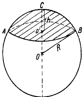
Calotă sferică
