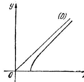
Asimptotă
