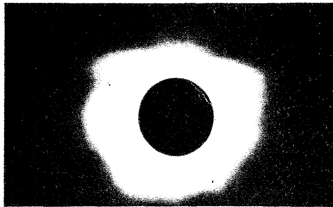
Coroana solară (fotografie făcută la București în timpul eclipsei din 15 februarie 1961)
