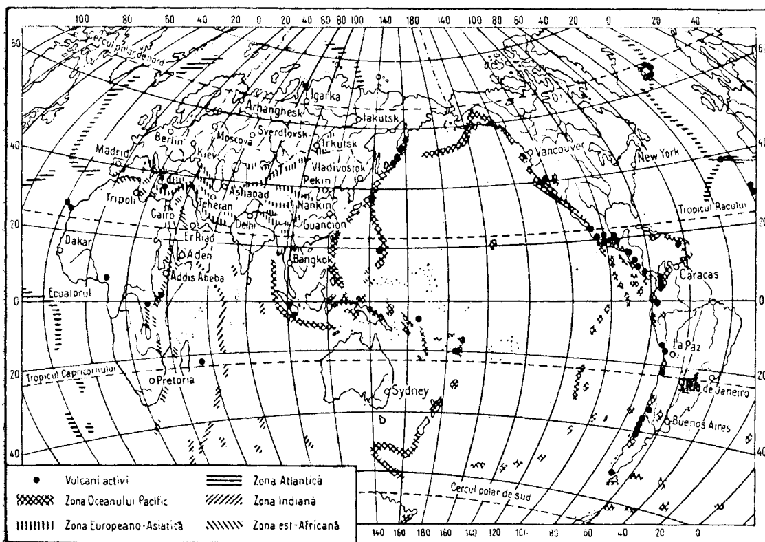
Răspândirea cutremurelor
