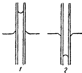
Capilaritate
