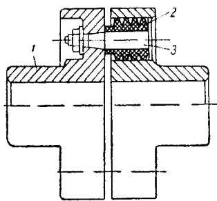
Cuplaj elastic
