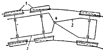
Schema înscrierii în curbă prin bisel 1 — osii fixe; 2 — lonjeron; 3 — cadrul triunghiular al biselului; 4 — pivot de rotație
