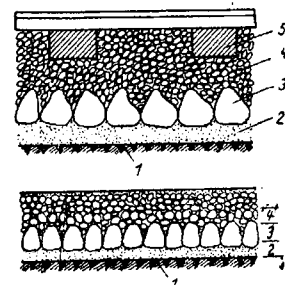
Blocăj sub balastul căilor ferate 1 — platforma căii; 2 — strat de nisip; 3 — blocăj; 4 — balast; 5 — traversă
