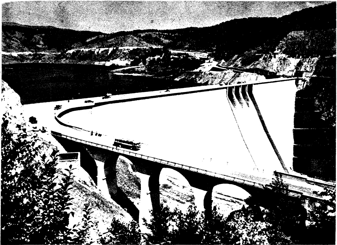
Barajul și lacul de acumulare al hidrocentralei
