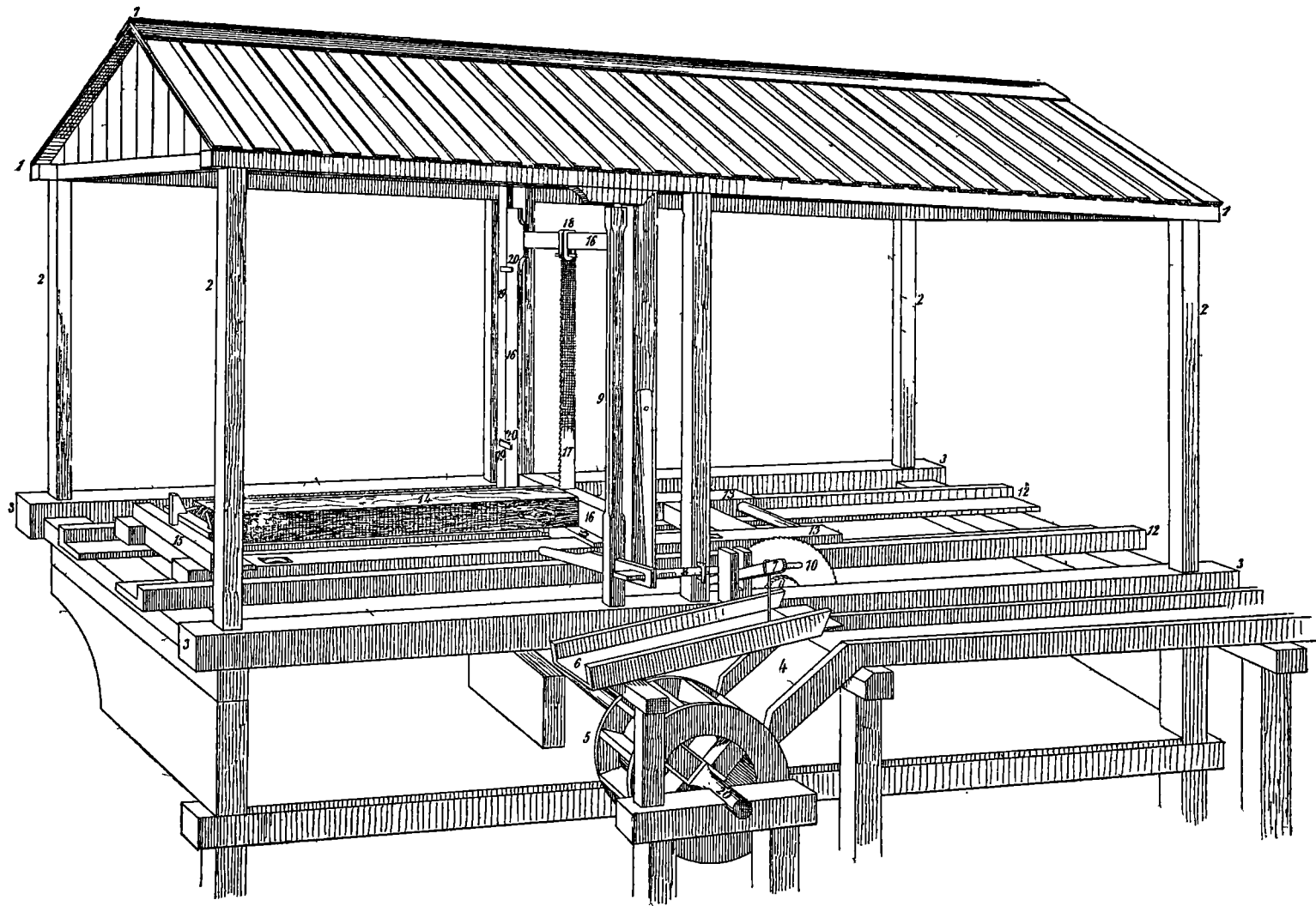
Fig. 2. Joagăr saŭ ferestreu de munte.
