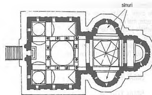
Biserica Mînăstirii Argeș, secțiune și plan
