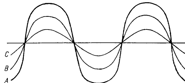
Fig. 4. — Vibrație compusă (A) din două vibrații cu aceeași frecvență și aceeași fază (B și C). (După B. Malmberg.)
