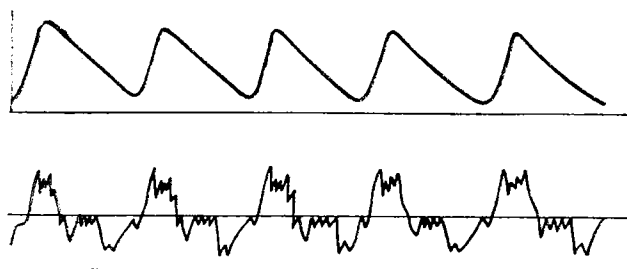
Fig. 5. — Curba tonului laringian (sus) înainte de producerea efectului rezonator al cavităților supraglotale și același ton (jos) după amplificarea anumitor armonice ale sale prin rezonanță. (După B. Malmberg.)
