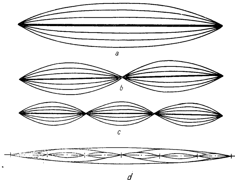
Fig. 3. — Originea tonurilor armonice. Vibrația coardei întregi (a), a jumătăților (b) și a treimilor (c). (După B. Malmberg.) Vibrația coardei (d). (După L. R. Zinder.)
