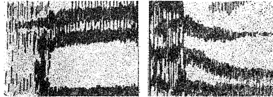
Fig. 10. — Spectrograma grupurilor si (stînga) și su (dreapta). Se vede că formantii vocalelor sînt deja net perceptibili în zgomotul consoanei precedente, care are o coloratură determinată de vocală. E vorba în realitate de doi s diferiți, unul cu coloratură de i , celălalt cu coloratură de u . (După B. Malmberg.)
