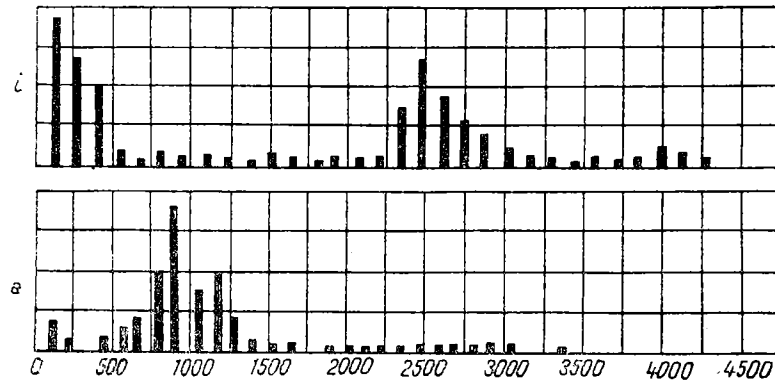
Fig. 6. — Spectrul vocalei i (sus) și al vocalei a (jos). (După B. Malmberg.)
