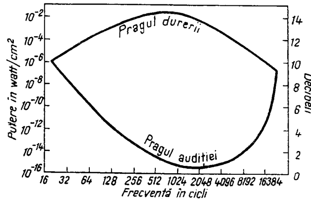
Fig. 2. — Cîmpul auditiv al omului. În abscisă, diferitele frecvențe, de la limita inferioară (16 p/s) pînă la limita superioară (circa 16 000 p/s); în ordonată, intensitatea fizică în wați pe \text{cm}^2 și cea subiectivă în decibeli. (După Al. Rosetti.)
