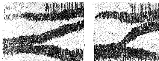
Fig. 8. — Spectrogramele diftongilor ai (la stînga) și oi (la dreapta) din limba engleză. Se vede cum trecerea de la primul element la al doilea se face succesiv. Formanții se îndepărtează din ce în ce mai mult unul de altul. Nu există un veritabil i decît spre sfîrșitul celui de-al doilea element. (După B. Malmberg.)
