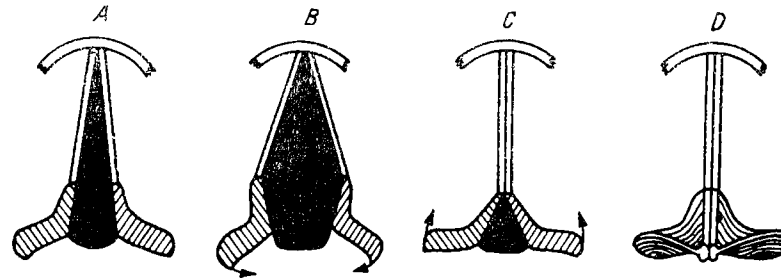
Fig. 12. — Glota. Coardele vocale sînt fixate în față (în figură — sus) de cartilajul tiroid, iar în spate (jos) de cartilajele aritenoidice, mobile. A : respirație normală; B : respirație profundă; C : graiul șoptit; D : poziția caracteristică pentru fonațiune. (După Al. Rosetti.)
