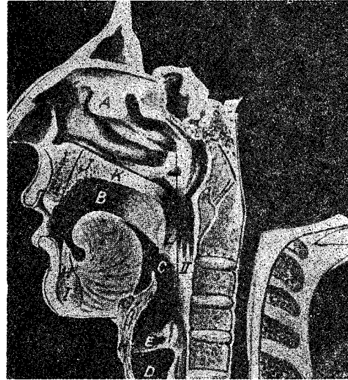
Fig. 11. — Organele vorbirii. Tăietură longitudinală. A. Cavitatea nazală. B. Cavitatea bucală. C. Faringele. D. Laringele. E. Glota. F. Muşchiul lingual (limba). G. Epiglota. H, H'. Dinţii. I. Maxilarul superior. I'. Maxilarul inferior. J. Palatul tare. K. Palatul moale (vălul palatului). L. Uvula. M. Cartilajul tiroid. (După Al. Rosetti.)
