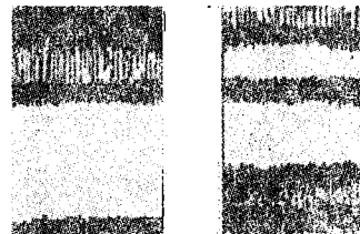
Fig. 8. — Spectrogramele diftongilor ai (la stînga) și oi (la dreapta) din limba engleză. Se vede cum trecerea de la primul element la al doilea se face succesiv. Formanții se îndepărtează din ce în ce mai mult unul de altul. Nu există un veritabil i decît spre sfîrșitul celui de-al doilea element. (După B. Malmberg.)
