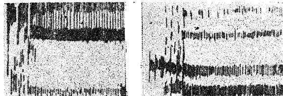
Fig. 9. — Spectrograma grupurilor ki (la stînga) și ku (la dreapta). Zgomotul consoanelor capătă pe spectrogramă formă de linii negre neregulate (la stînga pe figuri). Se vede net că zgomotul caracteristic al lui k se află mult mai sus pe scară în fața vocalei i (anterioară) decît în fața vocalei u (posterioară). E vorba în realitate de două fenomene acustice destul de diferite, deși urechea le identifică. (După B. Malmberg.)
