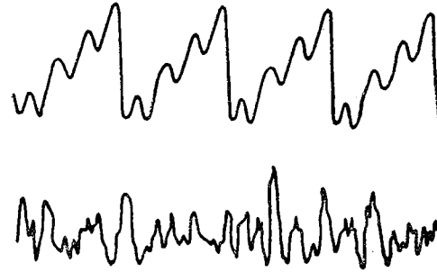
Fig. 1. — Curba unui sunet muzical (vibrații periodice) sus și a unui zgomot (vibrații neperiodice) jos. (După Al. Rosetti.)
