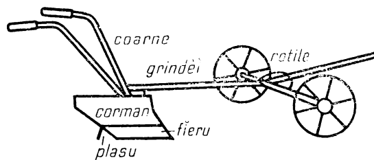
Părțile plugului (com. Dăbuleni)
